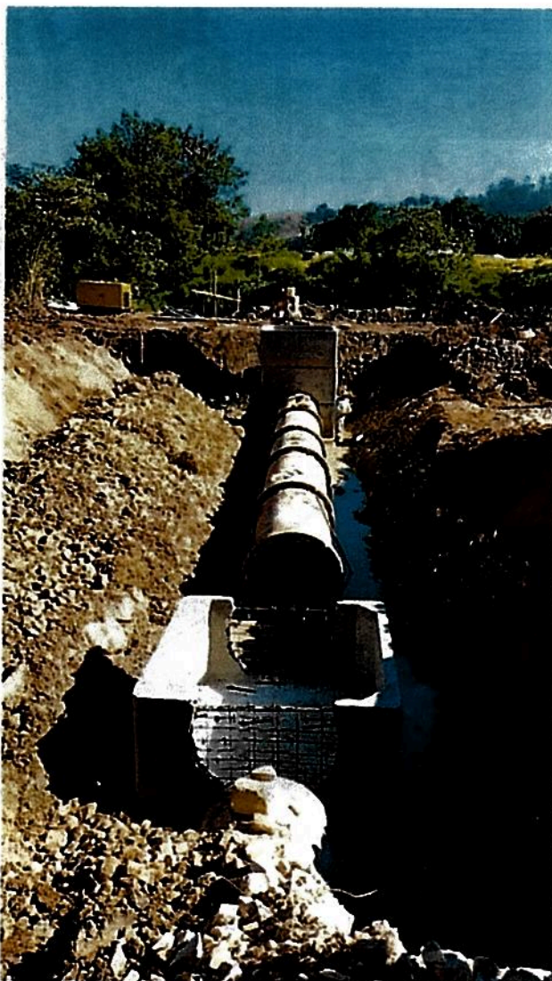
Figura 03 – Instalação dos tubos e PVs
